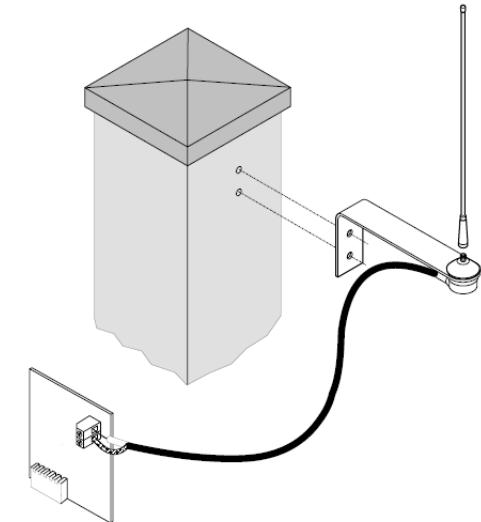
Монтаж выносной антенны
